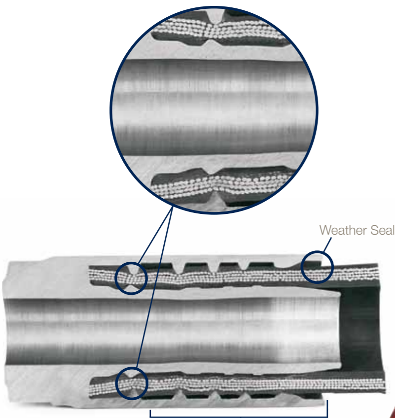
Kombinierte Interlock Verbindung mit zusätzlicher Haltekraft
